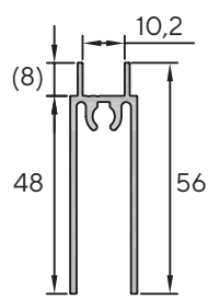
Profil orizontal inferior
