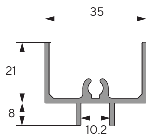
Profil orizontal superior
