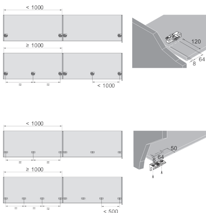
Vedere în secțiune a corpului de mobilier
