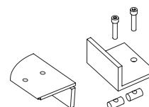
Opritor SAS 540.200
