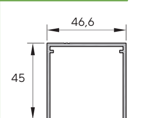
Șină superioară cu 1 cale
