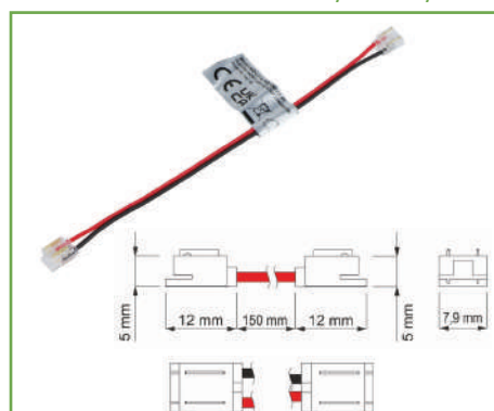
CABLU 0,15 M CU MICRO CONECTORI UNIVERSALI LA AMBELE CAPETE PENTRU BANDĂ LED COB/SMD 8/10 mm
