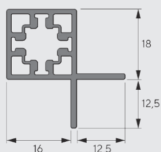
9303886 - montaj raft cu șuruburi
