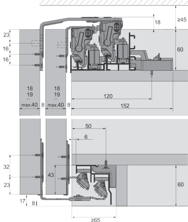
Dimensiuni montaj 2 uși
