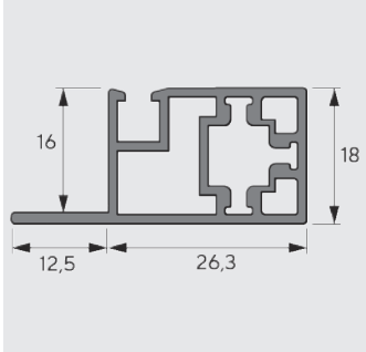
Montaj încadrat, profil inferior 9298804
