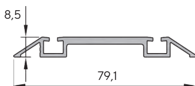
SAS 510.103.00 Șină inferioară cu 2 căi
