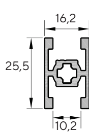
Profil divizor orizontal
