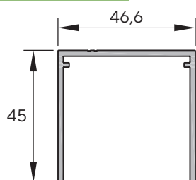
SAS 510.150.00 Șină superioară cu 1 cale
