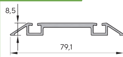
Șină inferioară cu 2 căi
