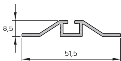
SAS 510.100.00 Șină inferioară cu 1 cale
