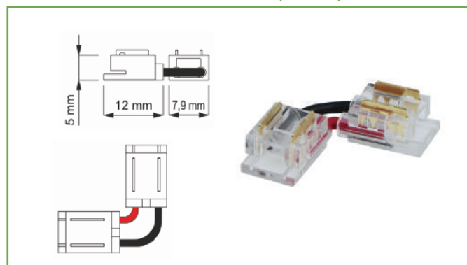
MICRO CONECTOR UNIVERSAL PENTRU ÎMBINARE ÎN UNGHI PENTRU BANDĂ LED COB/SMD 8/10 mm
