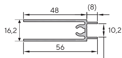
SAS 540.200 Set opritori superiori
