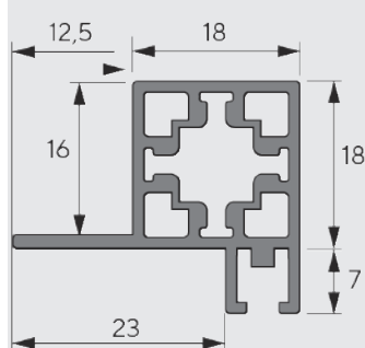
Montaj încadrat, profil superior 9298802
