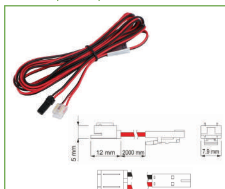
MICRO CONECTOR UNIVERSAL CU MINIMUFĂ, CABLU 2 M, PENTRU BANDĂ LED COB/SMD 8/10 mm
