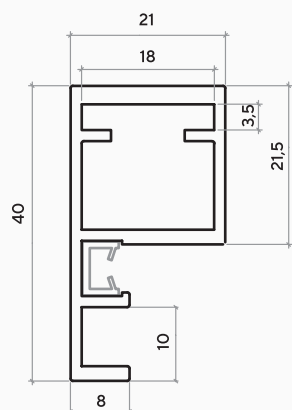
Profil mâner: HH165.003.001
