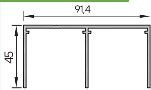
Șină superioară cu 2 căi
