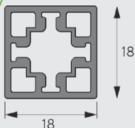
9303886 - montaj raft cu șuruburi
