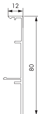
SAS 110.100 Profil de acoperire
