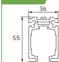
SAS 210.161 Cale de rulare
