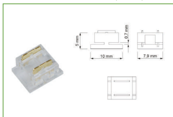
MICRO CONECTOR UNIVERSAL FĂRĂ FIRE PENTRU DOUĂ BENZI LED COB/SMD 8/10 mm
