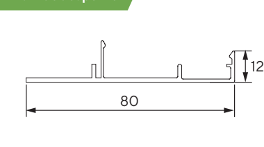
SAS 110.100 Profil de acoperire
