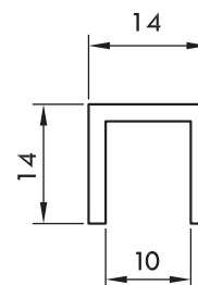
SAS 210.100.00 Profil de ghidaj
