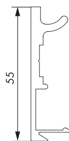
SAS 110.110 Profil montaj perete
