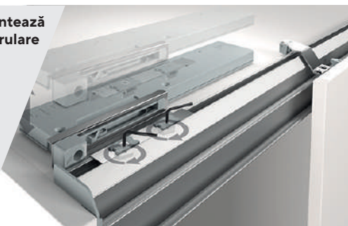
Profile de rulare și ghidare
