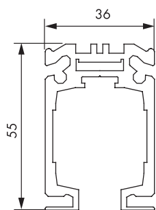
SAS 210.161 Cale de rulare
