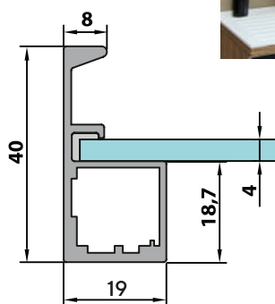
SAS 999H cu profil mâner
