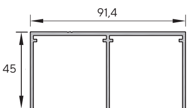
SAS 510.151.00 Șină superioară cu 2 căi
