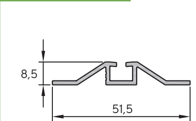
Șină inferioară cu 1 cale
