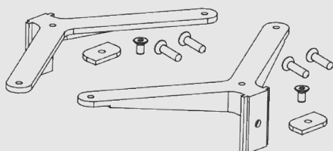
Set prindere polițe din lemn
