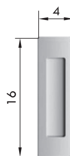
SAS 590.450.00 Mâner încastat
