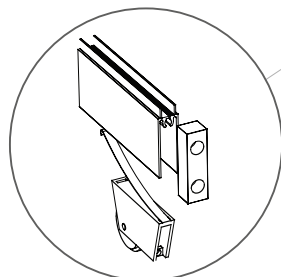
Role inferioare
